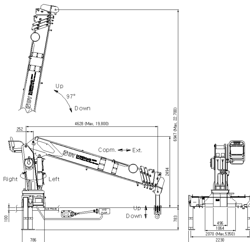
Рис. 3 КМУ модели SS1966 ACE. Схема общего вида.
