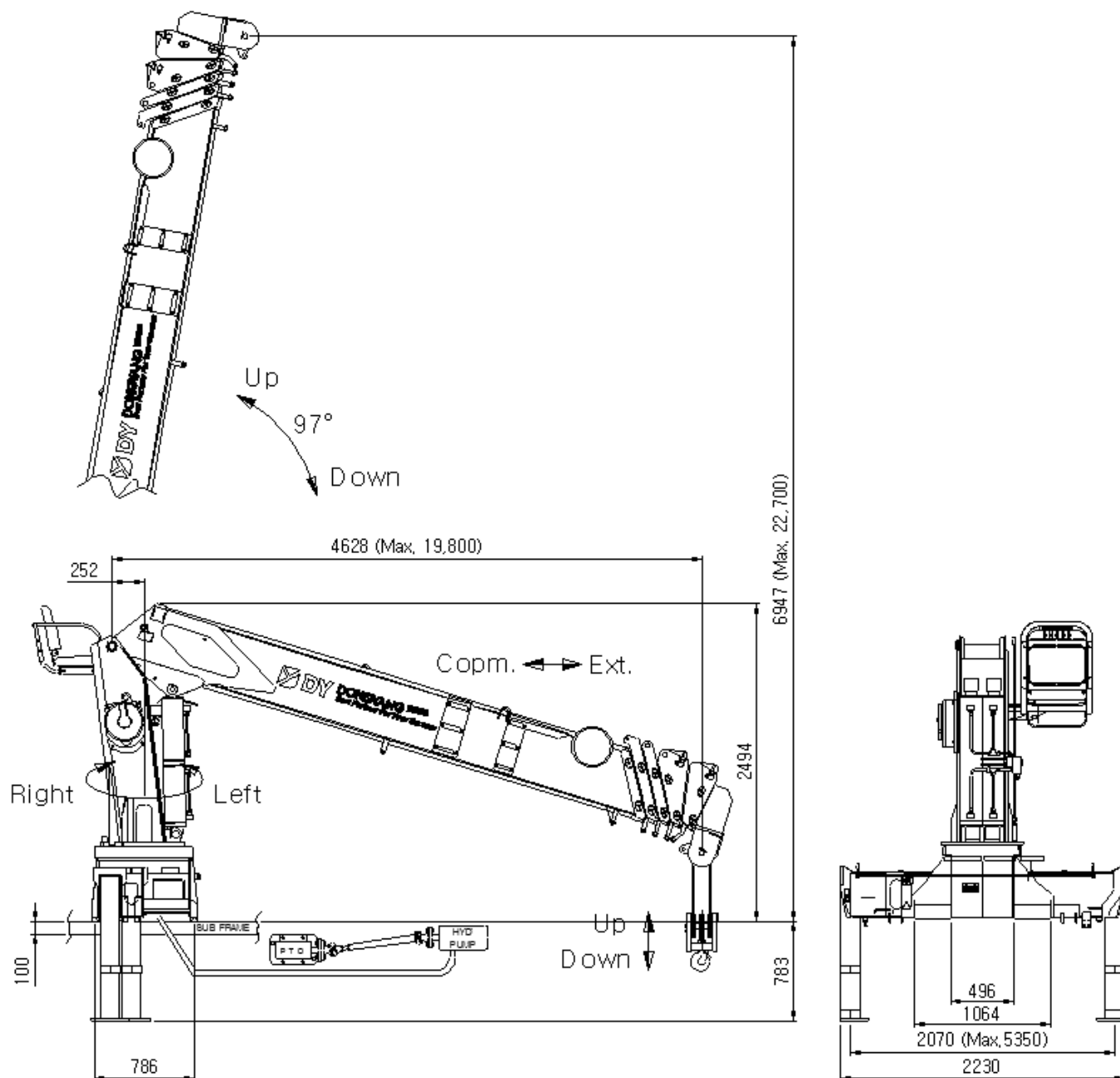
Рис. 1 Краноманипуляторная установка (КМУ) модели SM1966 ACE в рабочем положении.
