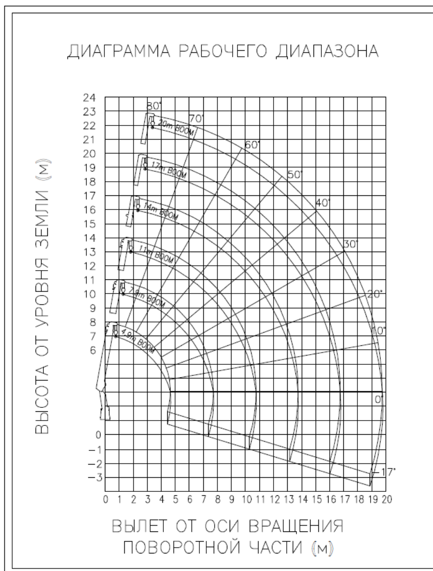
Рис. 2 Диаграмма высотных характеристик КМУ модели SS1966 ACE
